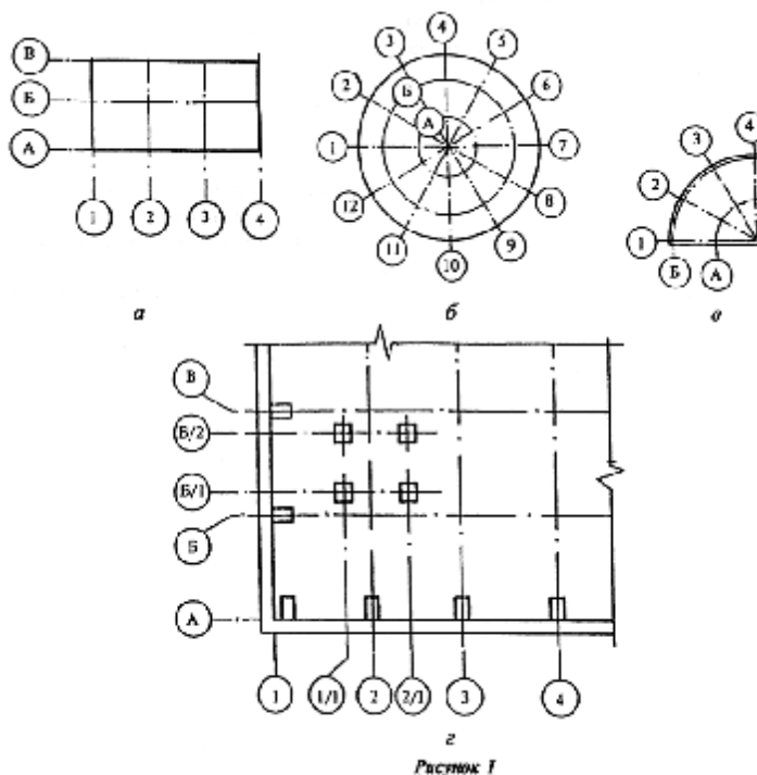
"Рисунок 1. Последовательность цифровых и буквенных обозначений координационных осей"
